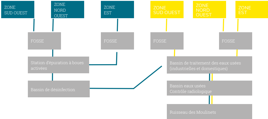
Schéma de collecte des eaux usées
