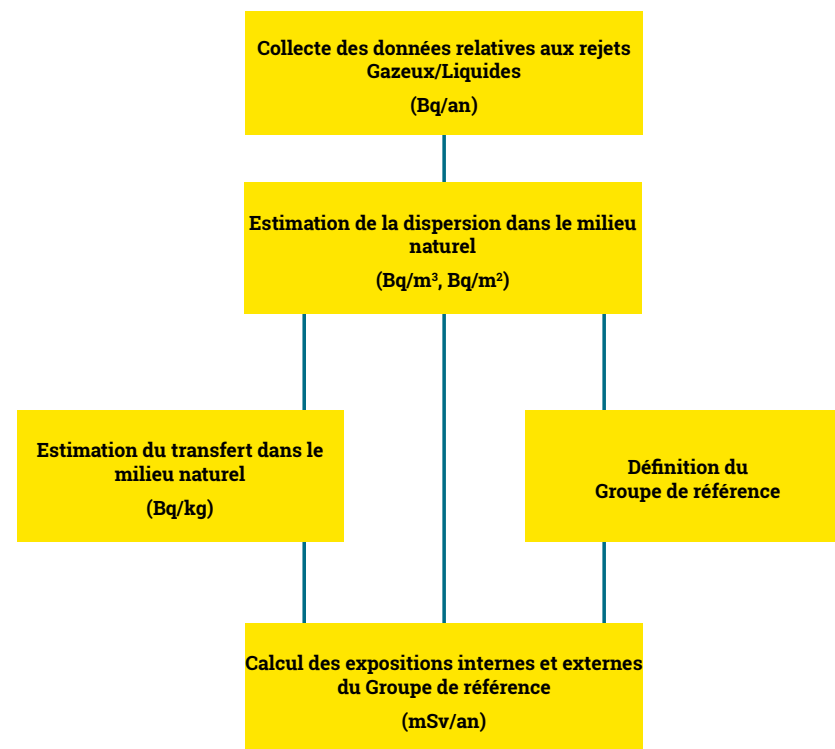
Schéma général du calcul d'impact
